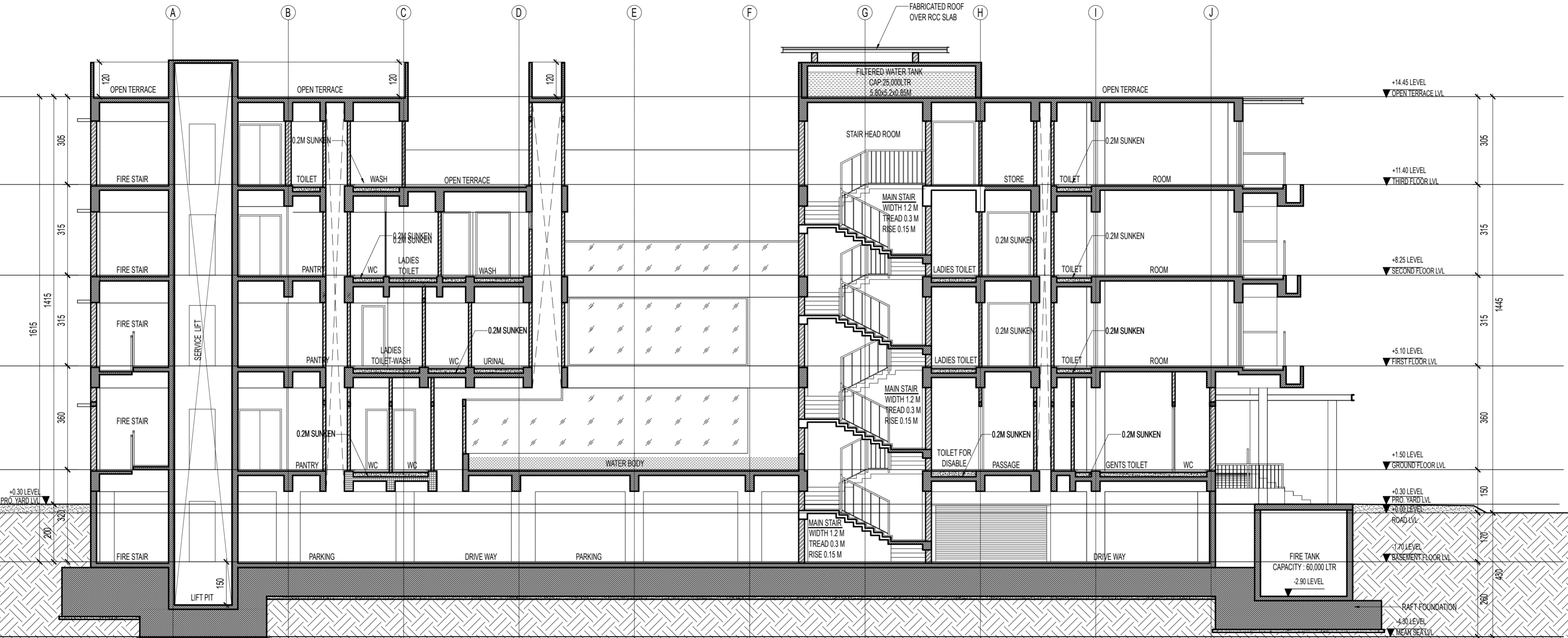
SECTION A-A SCALE 1:100
